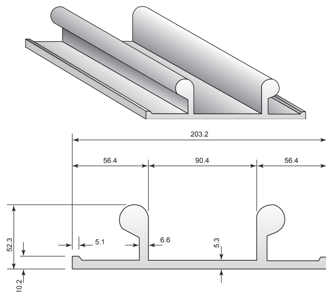
Corte transversal del riel vertical de alta resistencia
