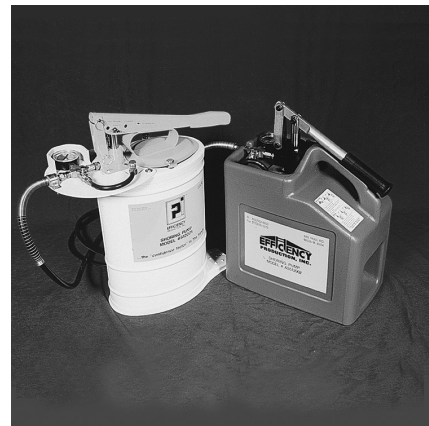
Bidón metálico de la bomba de 22,73 l (5 gal) (izquierda) y bidón plástico de la bomba de 22,73 l (5 gal) (derecha).
